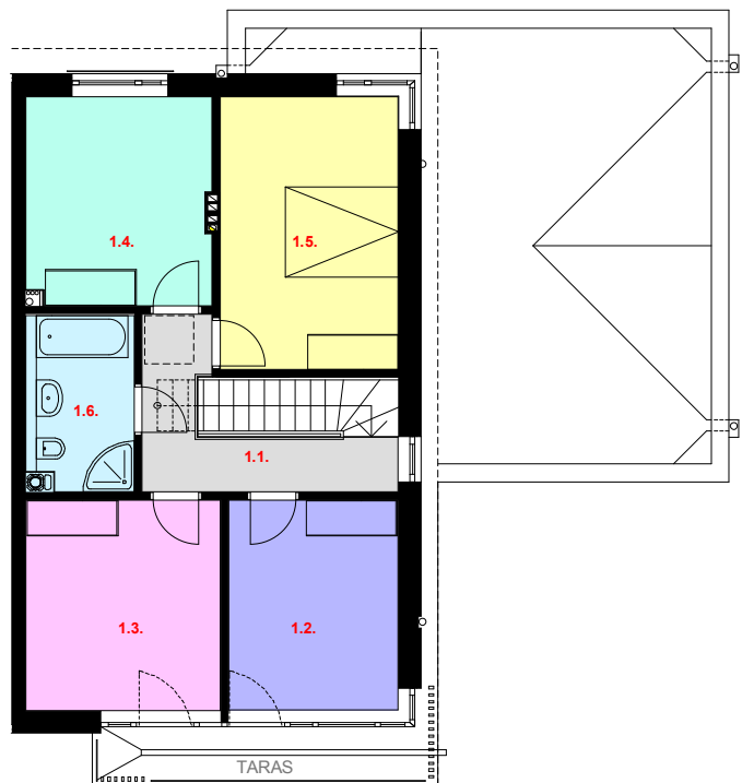
RZUT PIĘTRA
